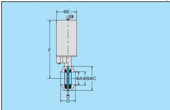
焊式气动防混蝶阀
