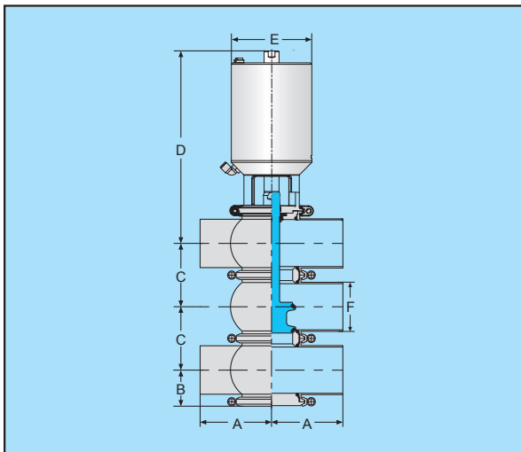
N型气动换向阀
