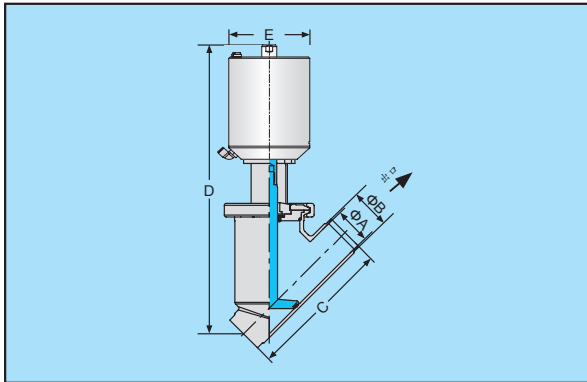
Y型手动截止阀
