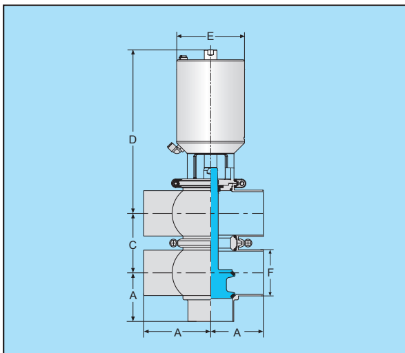
TT型气动换向阀
