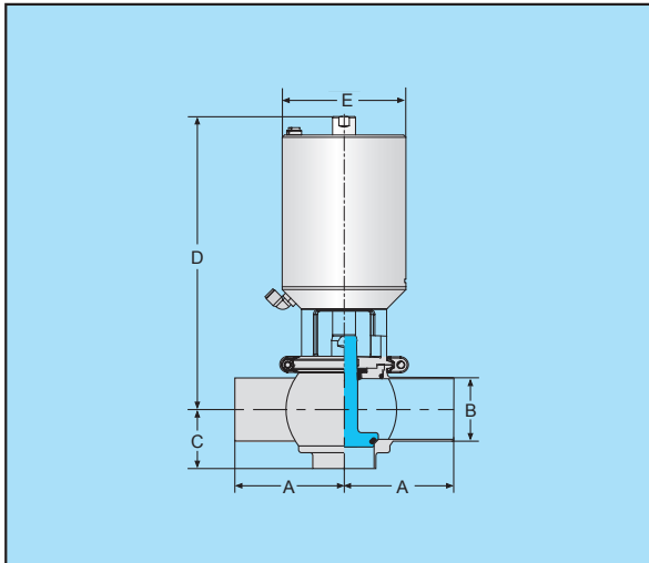
T型气动单座阀 (短型)
