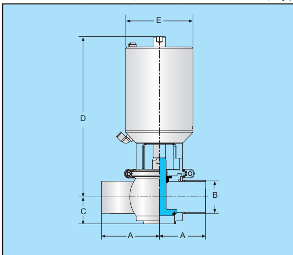
T型气动截止阀 (短型)
