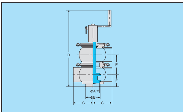
TT型手动换向阀 (短型)
