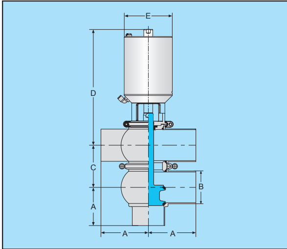
TL型气动换向阀
