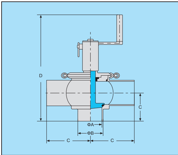
T型手动截止阀
