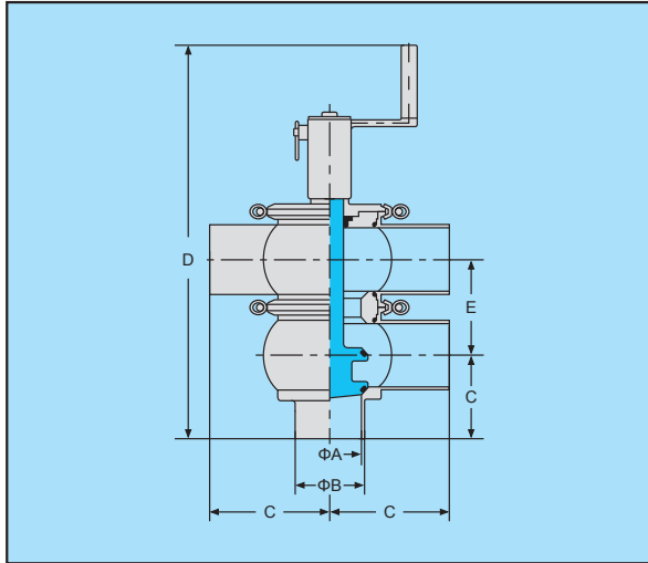
TL型手动换向阀
