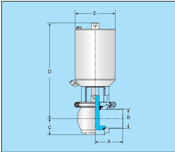
L型气动截止阀 (短型)
