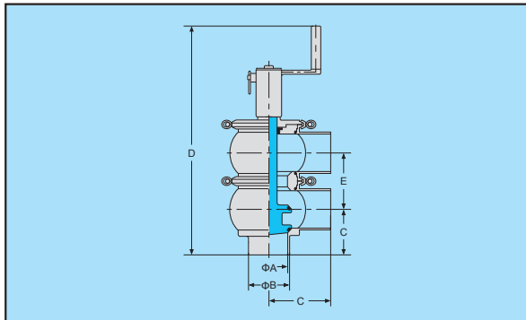
TL型手动换向阀
