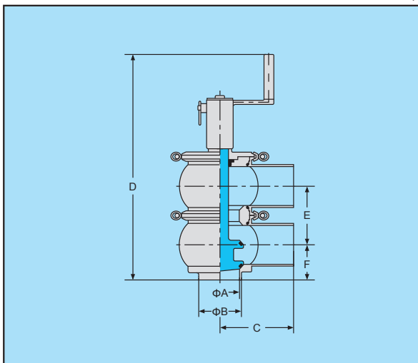
LL型手动换向阀 (短型)
