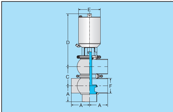
LT型气动换向阀
