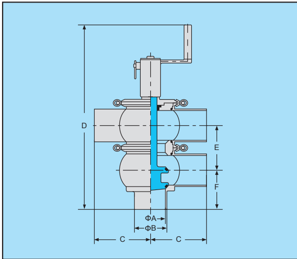
TL型手动换向阀 (短型)
