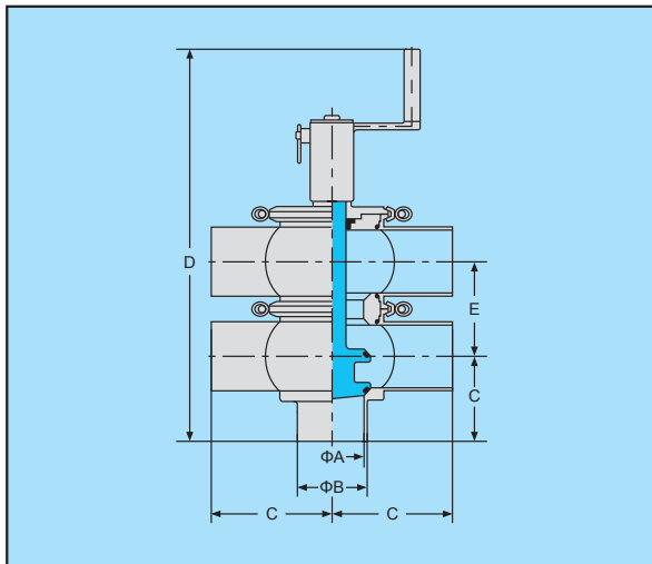
TT型手动换向阀
