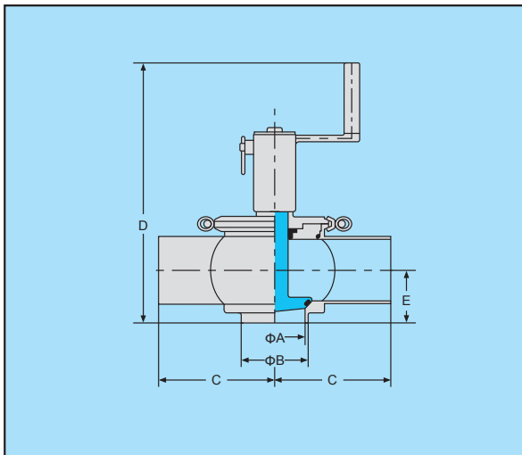
T型手动截止阀 (短型)
