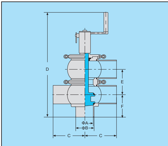
LT型手动换向阀 (短型)
