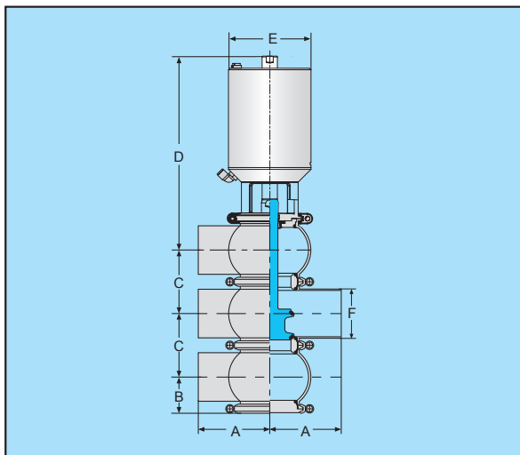
N型气动换向阀
