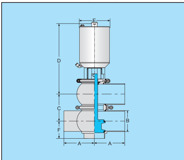
LT型气动换向阀 (短型)
