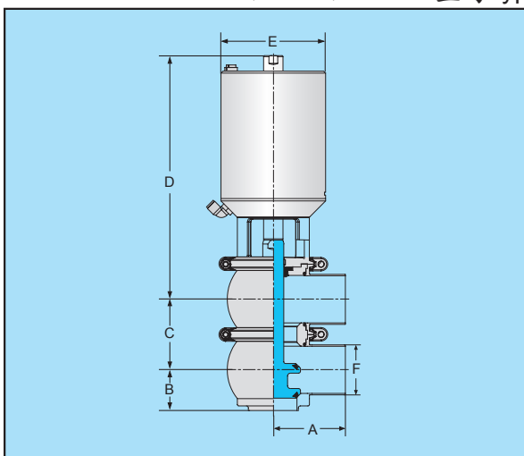
LL型气动换向阀 (短型)
