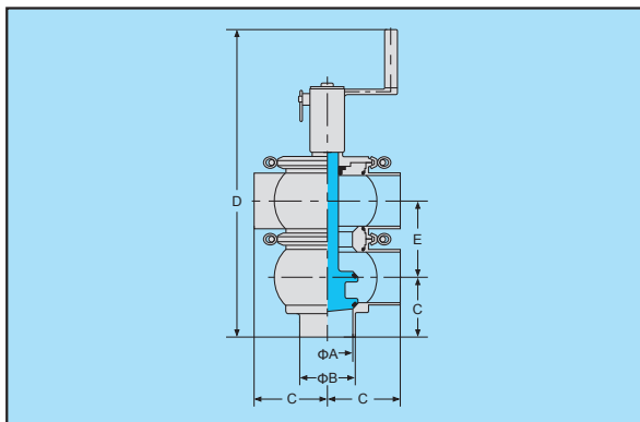
TL型手动换向阀
