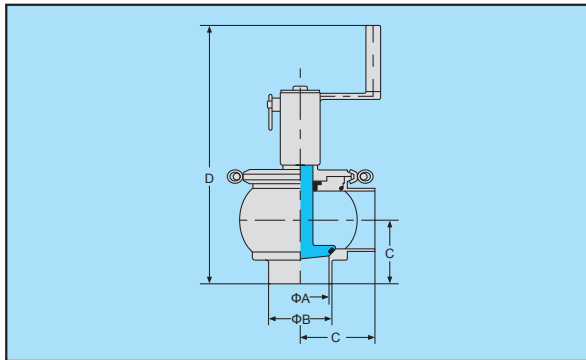
T型手动截止阀
