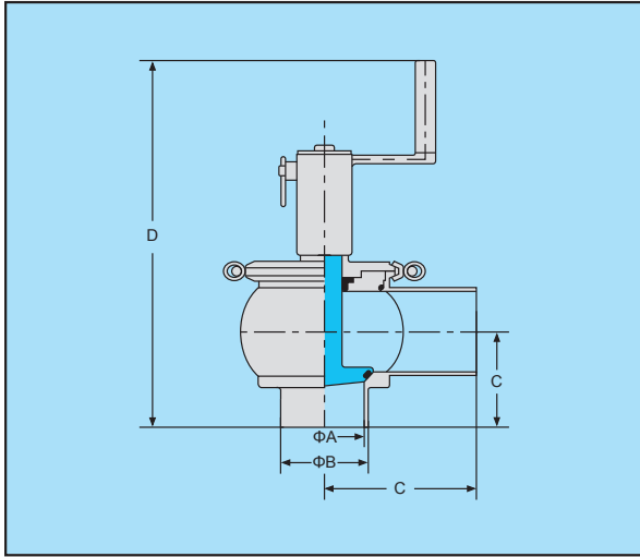
L型手动截止阀
