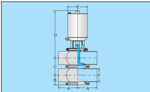
LL型气动换向阀
