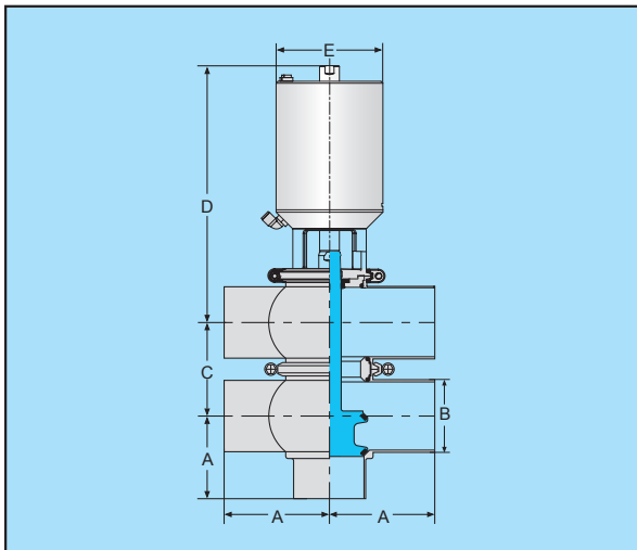
TT型气动换向阀
