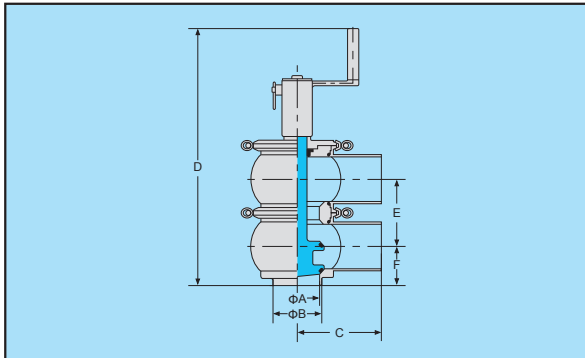
TL型手动换向阀 (短型)
