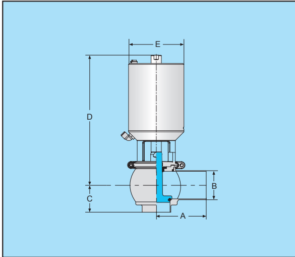
L型气动单座阀 (短型)
