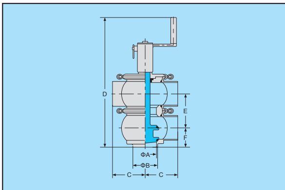
TL型手动换向阀 (短型)
