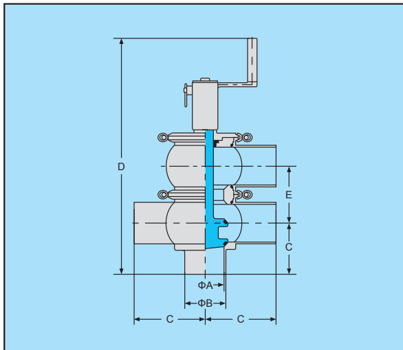
LT型手动换向阀
