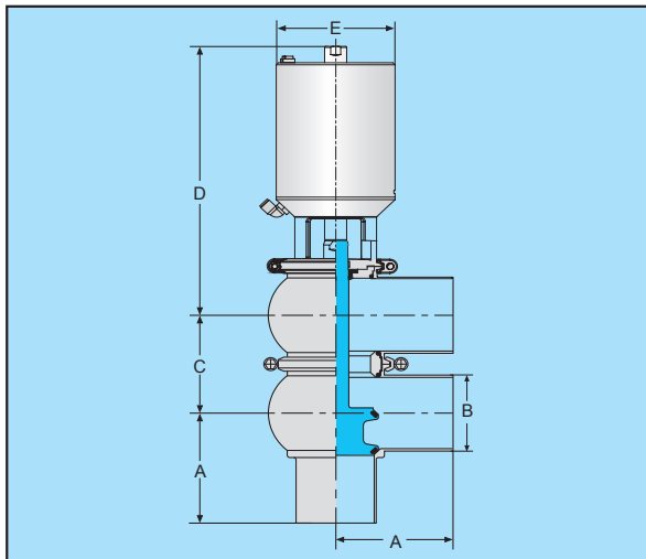
LL型气动换向阀
