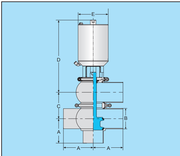
LT型气动换向阀
