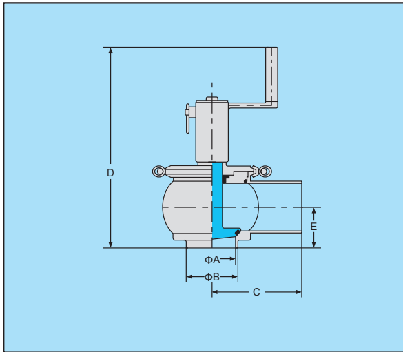
L型手动截止阀 (短型)
