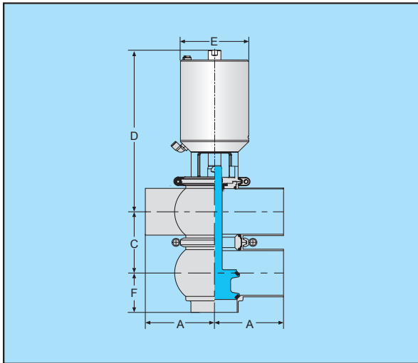
TL型气动换向阀 (短型)
