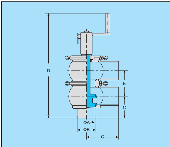
LL型手动换向阀
