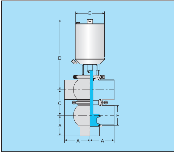
TL型气动换向阀
