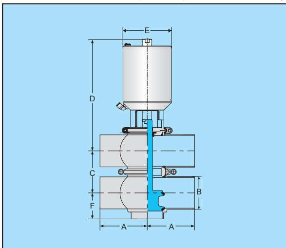
TT型气动换向阀 (短型)
