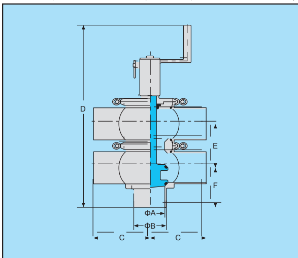
TT型手动换向阀 (短型)
